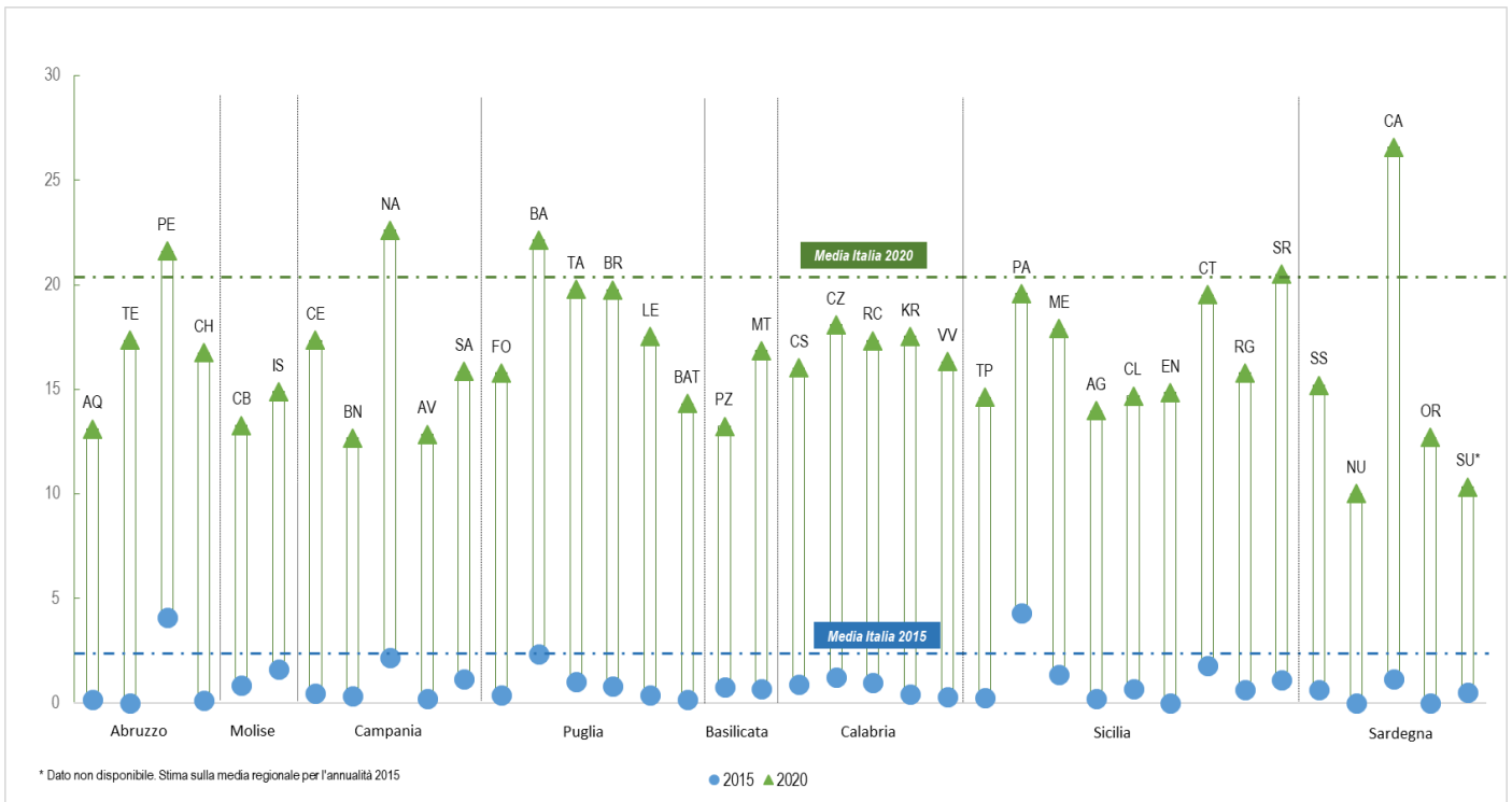
Figura 5.1 - Penetrazione della banda ultra larga. Province del Mezzogiorno. Anni 2015, 2020 e relative tendenze (valori %)
