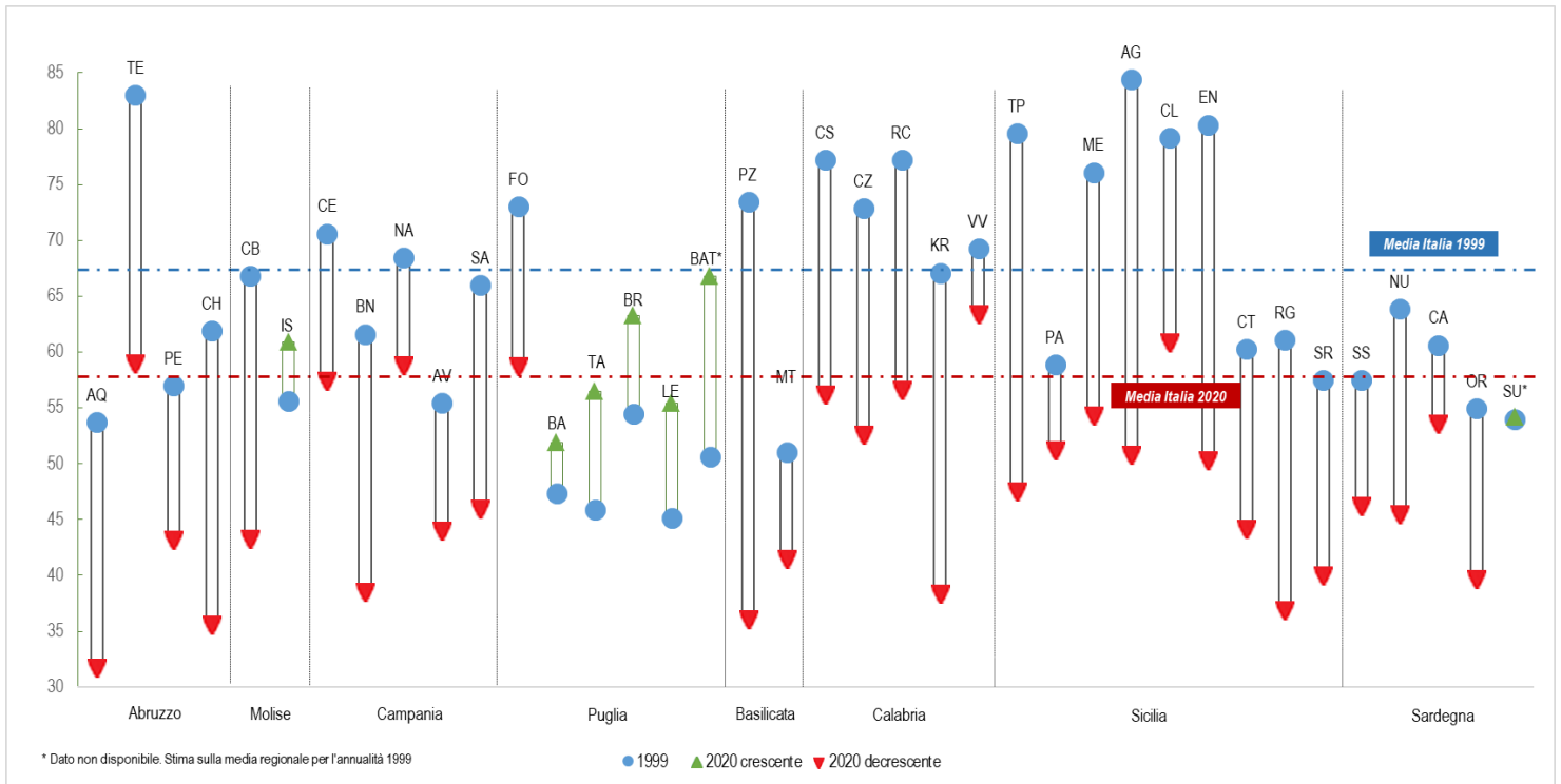
Figura 6.1 - Efficienza reti idriche. Province del Mezzogiorno. Anni 1999, 2020 e relative tendenze (valori %)
